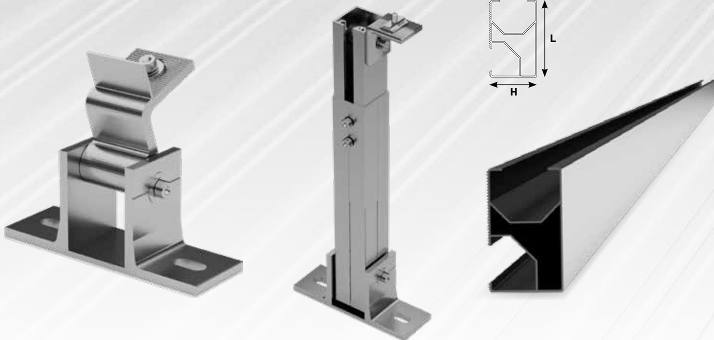
FS-AD APOIO DIANTEIRO AJUSTÁVEL
