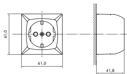
TOMADA COM CAIXA
